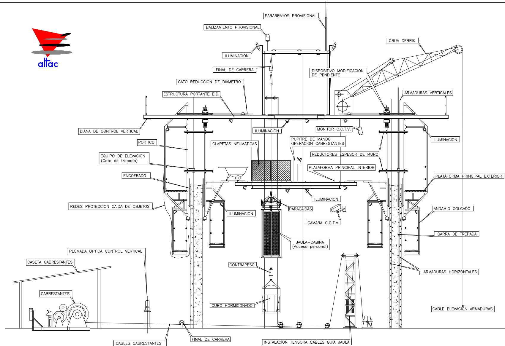
SISTEMA DE ENCOFRADO DESLIZANTE
